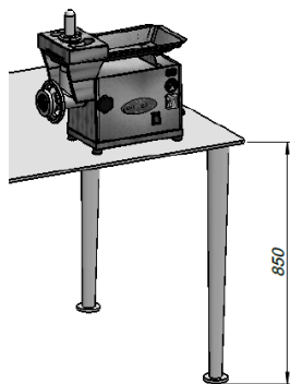
Fig. 5 – Altura bancada
