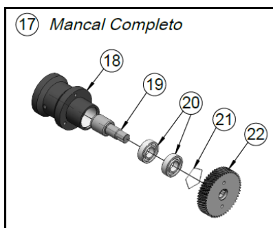
Fig. 3 – Componentes de reposição – Mancal Completo
