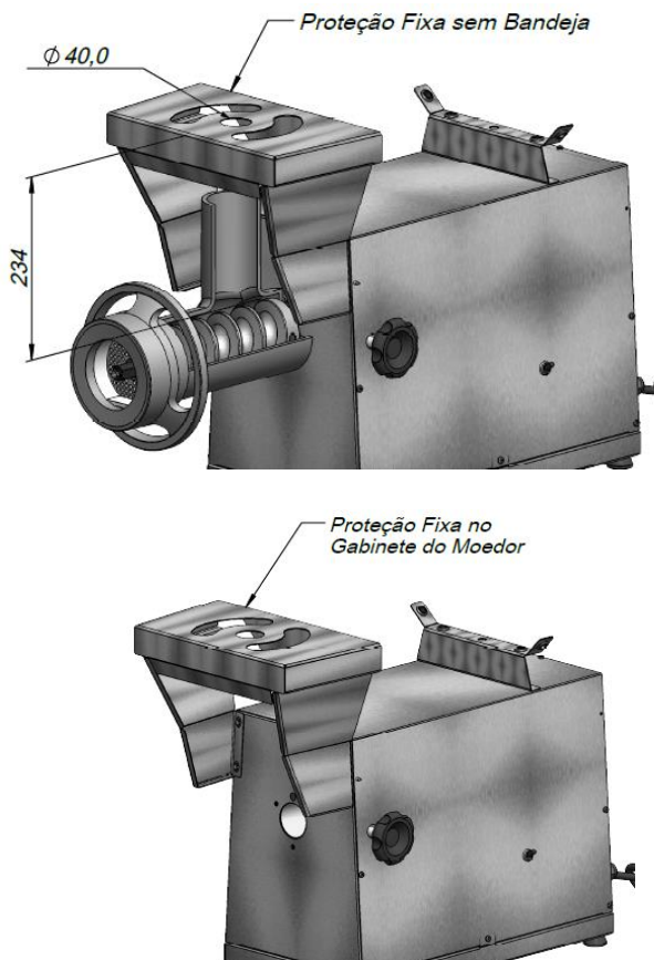
Fig.9- impedindo o ingresso dos membros superiores na zona da rosca sem fim – ITEM ATENDIDO
