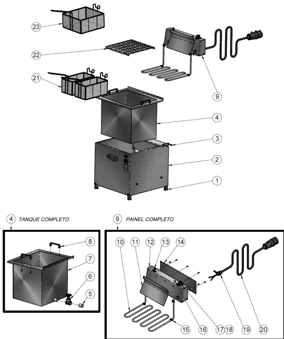
Fig. 1 – Componentes de reposição
