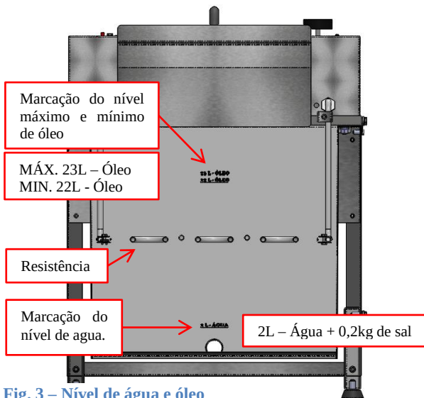
Fig. 3 – Nível de água e óleo
